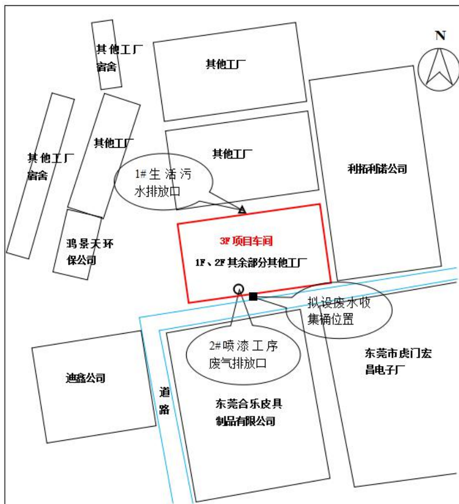
图3-1 厂区平面布置及监测点位
