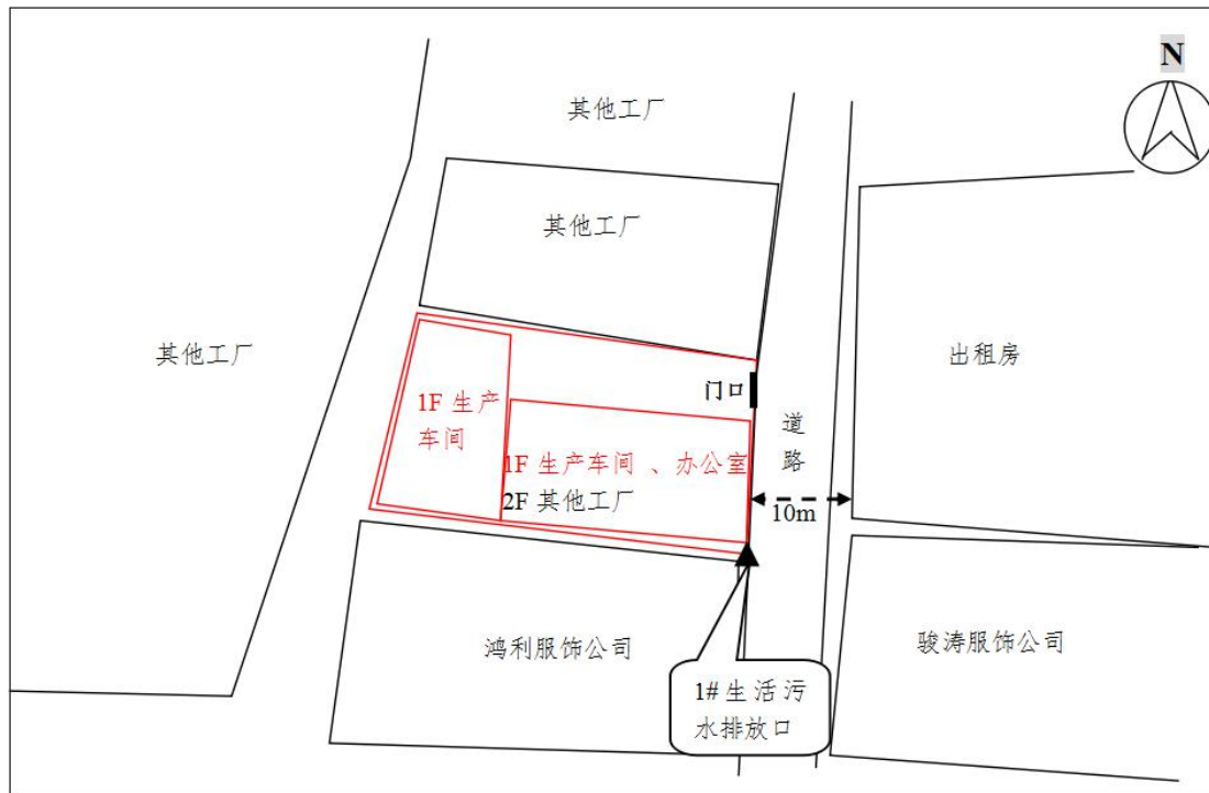
图3-1 厂区平面布置及监测点位
