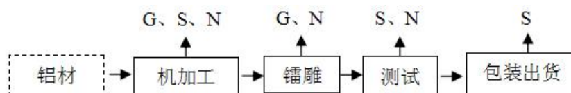
图 3-3 项目手机配件生产工艺及产污环节流程图
