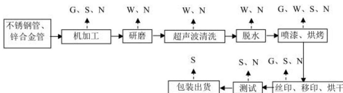
图 3-2 不锈钢管、锌合金管生产工艺及产污环节图
