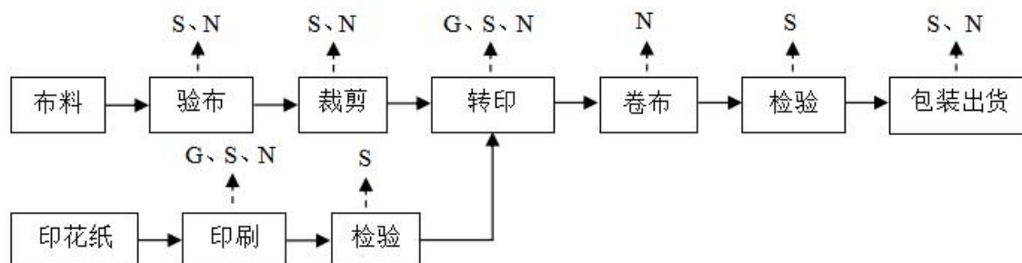
图 3-2 印花布生产工艺及产污环节图
