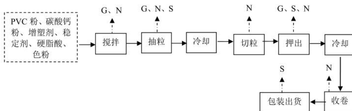
图 3-3 项目电线生产工艺及产污环节流程图
