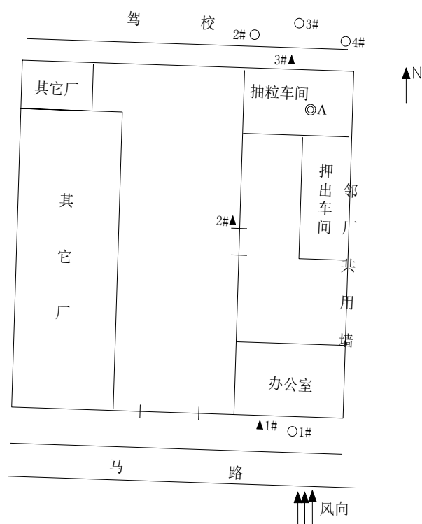
图 3-2 厂区平面布置及监测点位
