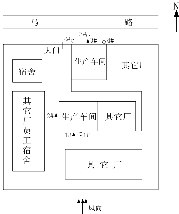
图 3-2 厂区平面布置及监测点位
