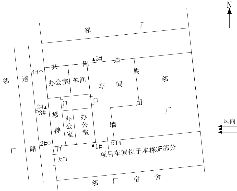
图 3-2 厂区平面布置及监测点位
