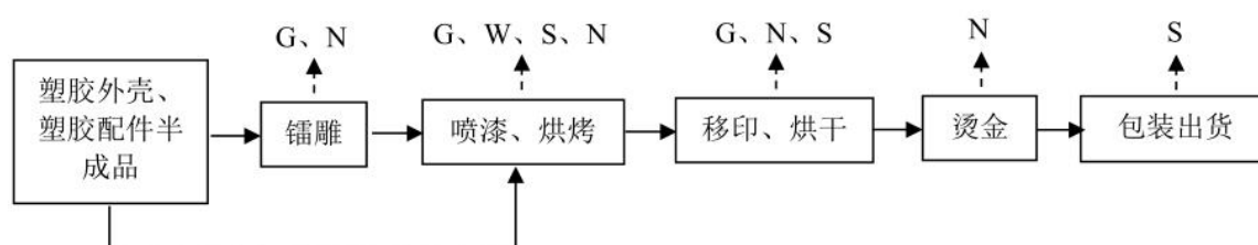
图 3-2 塑胶外壳、塑胶配件生产工艺及产污环节图
