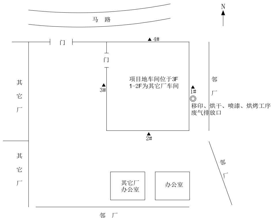
图 3-1 厂区平面布置及监测点位
