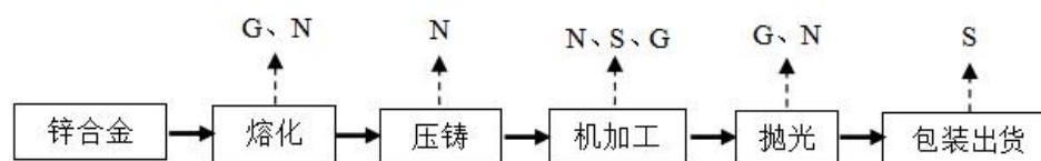
图 3-3 项目生产工艺及产污环节流程图
