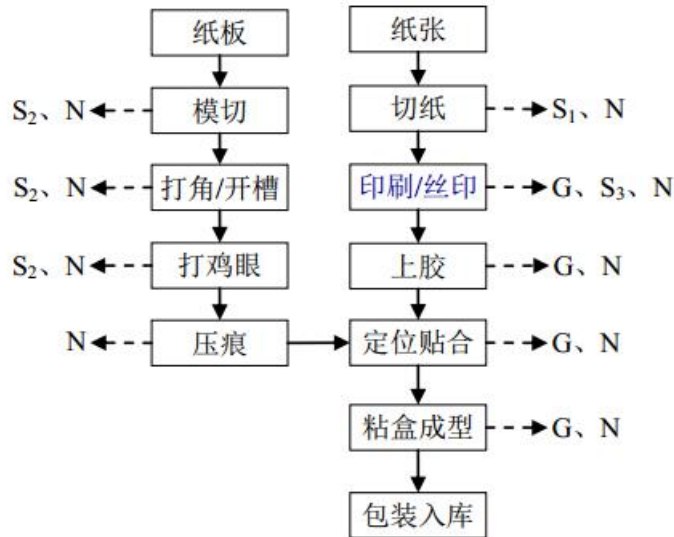
图 3-3 彩盒生产工艺及产污环节流程图
